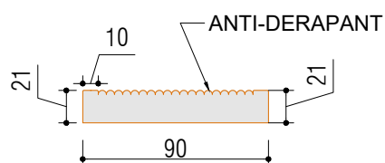
DECKING ANTI-DERAPANT - COUPE
