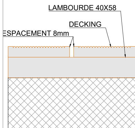
VUE DE COUPE
