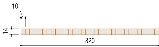
PARQUET INDUSTRIEL - COUPE
