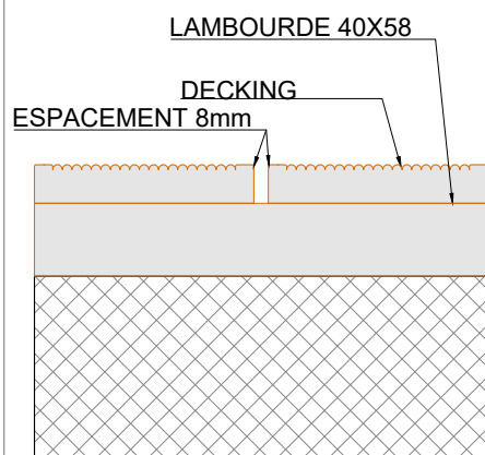
VUE DE COUPE
